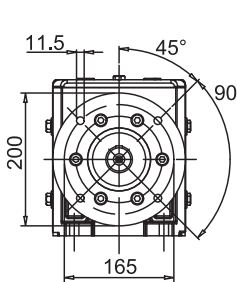
Eingebauter Flansch Flange modular
