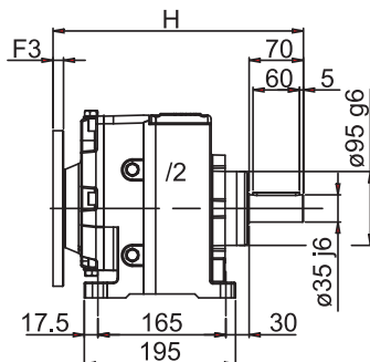
Eingebauter Flansch Flange modular
