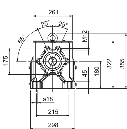
Flangia Riportata Bride modulaire
