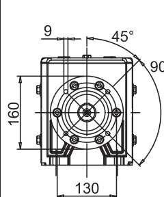
Flangia Riportata Bride modulaire
