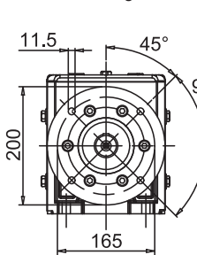
Eingebauter Flansch Flange modular
