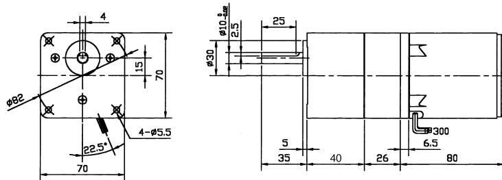
Fig.3 GEARED MOTOR WITH DECIMAL GEAR (中間 GEAR 使用時) WT 1.2 + 0.5/0.6 + 0.25 kg IH7PF15 + 7H10X + 7H □ FM (7H □ FB)
