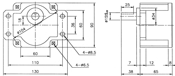
Fig.3 GEARED MOTOR WITH DECIMAL GEAR(中間 GEAR 使用時) IH9PF90 + 9H10X + 9H □ FM (9H □ FB)
